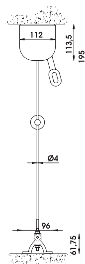
Držiak lanka do podlahy
