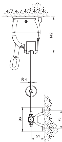
Montáž do stropu
