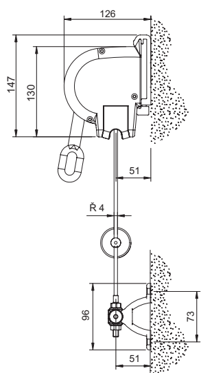
Držiak lanka na stenu
